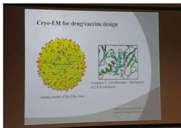
在冷凍電子顯微鏡下的寨卡病毒
