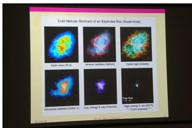
利用不同的天體望遠鏡觀察我們的天空
